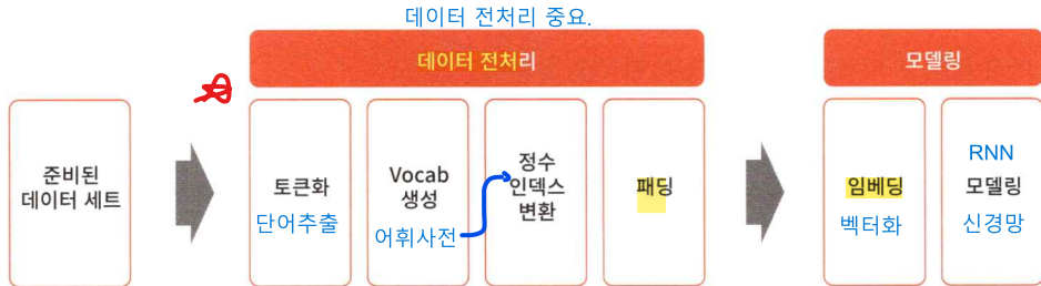
[그림 9-5] 언어 모델링 절차
